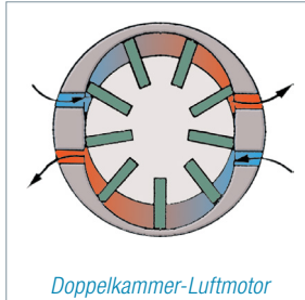
Doppelkammer-Luftmotor
